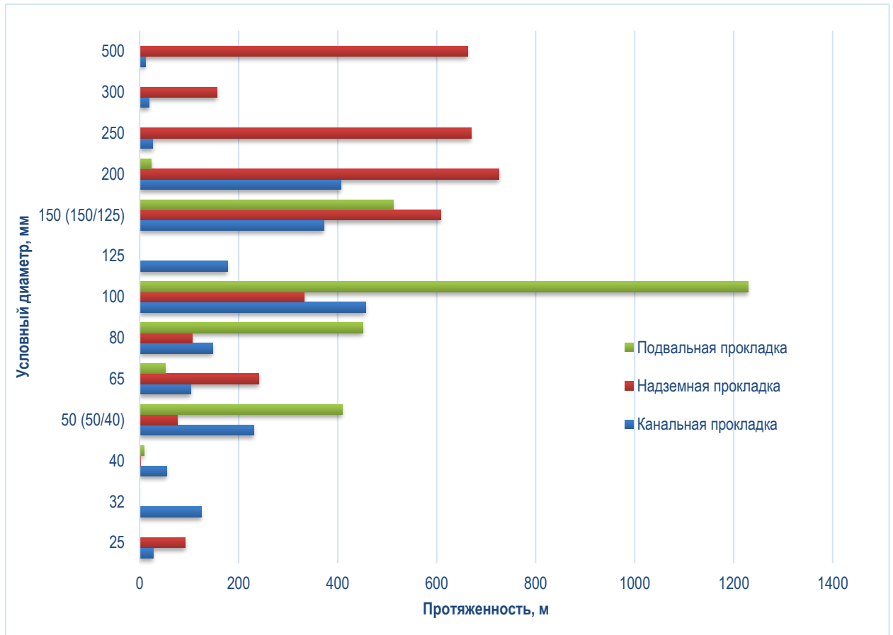
Рисунок 1.5 – Структура сетей отопления котельной п. Зональная Станция
